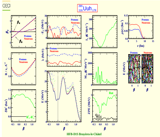
Ununhexium 295 (Z=116, N=179)
