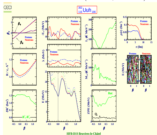
Ununhexium 302 (Z=116, N=186)
