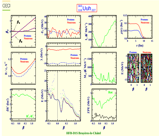
Ununhexium 343 (Z=116, N=227)
