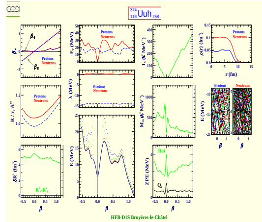
Ununhexium 374 (Z=116, N=258)
