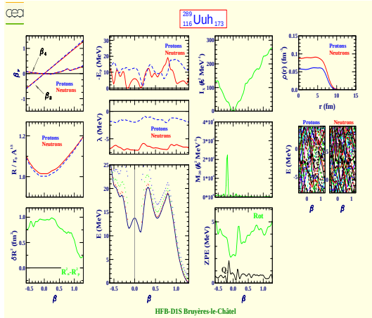
Ununhexium 289 (Z=116, N=173)
