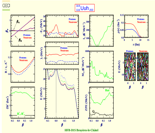
Ununhexium 319 (Z=116, N=203)
