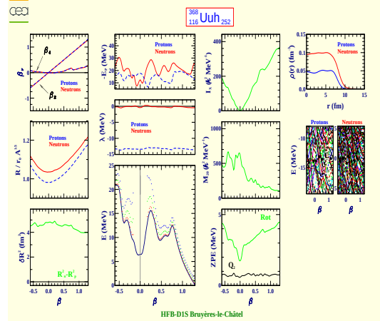
Ununhexium 368 (Z=116, N=252)
