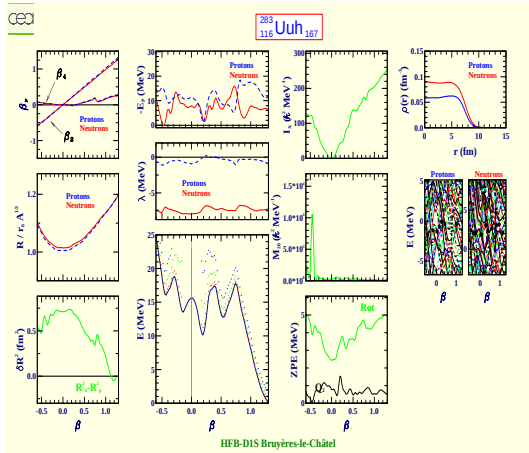
Ununhexium 283 (Z=116, N=167)
