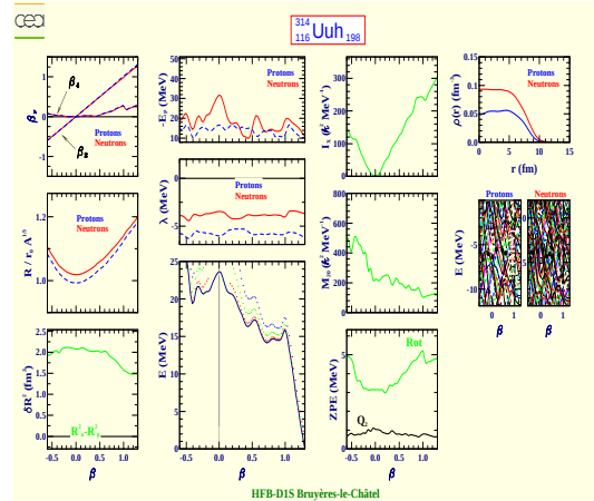
Ununhexium 314 (Z=116, N=198)
