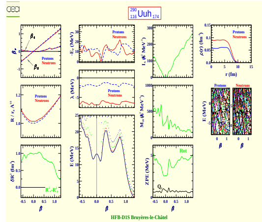
Ununhexium 290 (Z=116, N=174)
