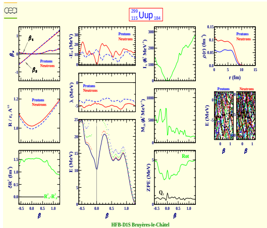
Ununpentium 299 (Z=115, N=184)
