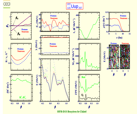
Ununpentium 372 (Z=115, N=257)
