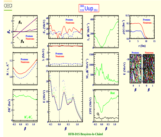
Ununpentium 366 (Z=115, N=251)
