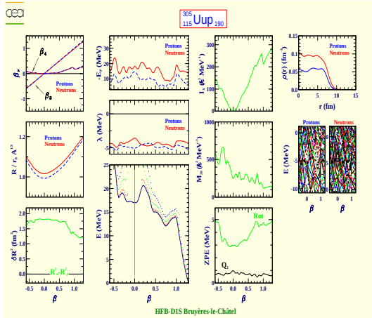
Ununpentium 305 (Z=115, N=190)
