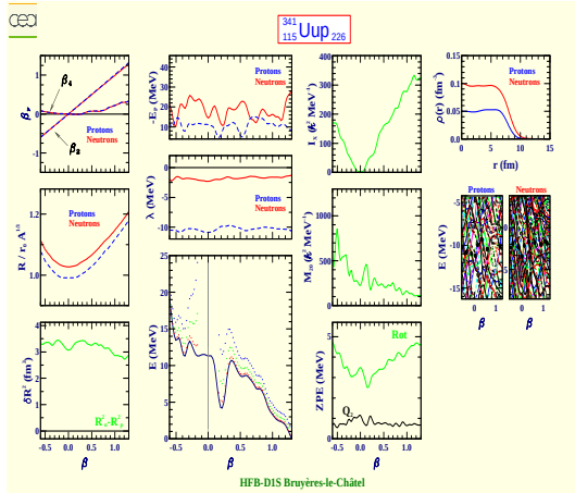
Ununpentium 341 (Z=115, N=226)
