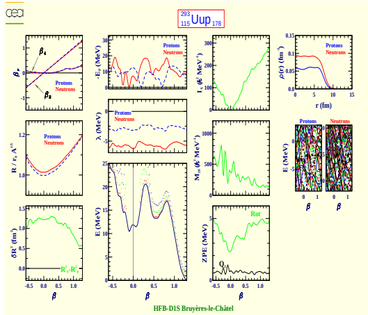
Ununpentium 293 (Z=115, N=178)
