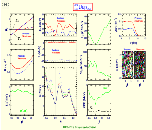
Ununpentium 371 (Z=115, N=256)
