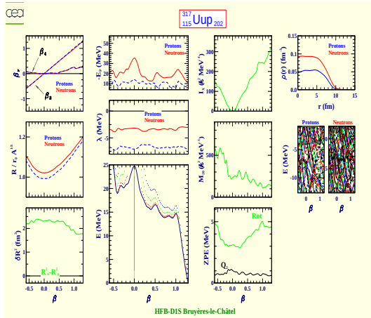
Ununpentium 317 (Z=115, N=202)
