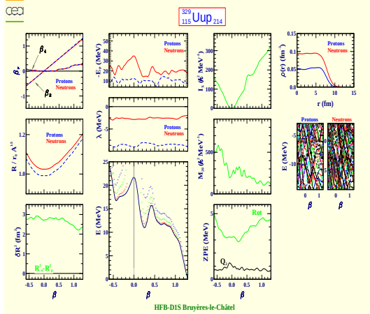
Ununpentium 329 (Z=115, N=214)
