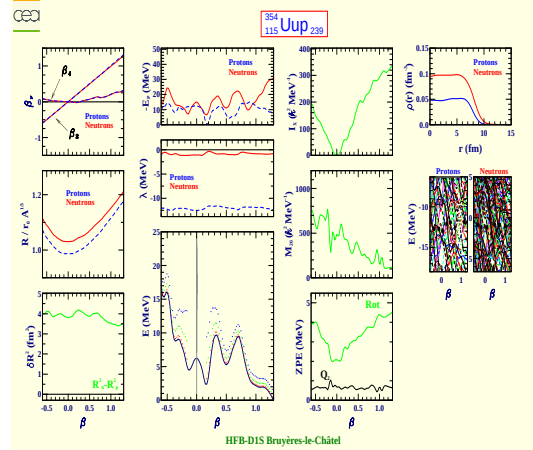
Ununpentium 354 (Z=115, N=239)
