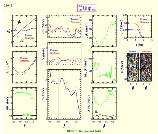
Ununpentium 306 (Z=115, N=191)
