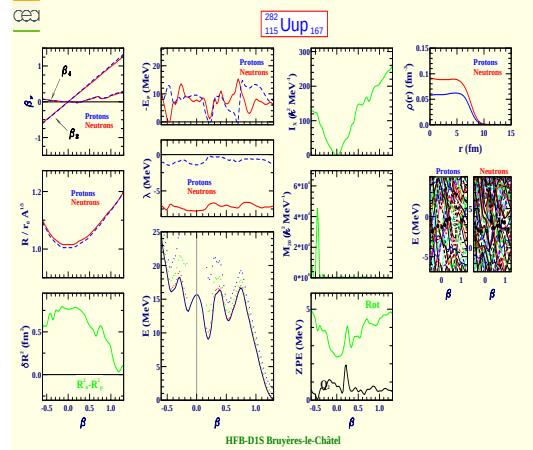
Ununpentium 282 (Z=115, N=167)
