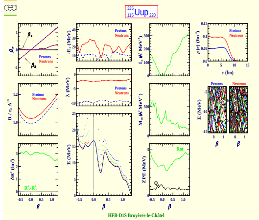
Ununpentium 335 (Z=115, N=220)
