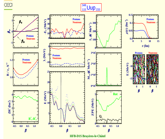
Ununpentium 348 (Z=115, N=233)
