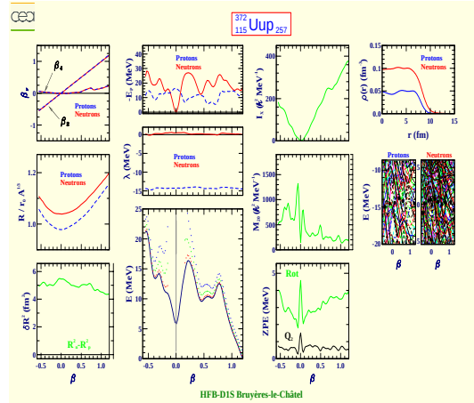
Ununpentium 372 (Z=115, N=257)
