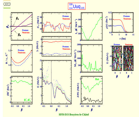
Ununquadium 339 (Z=114, N=225)
