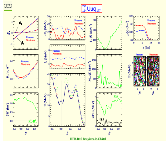
Ununquadium 291 (Z=114, N=177)
