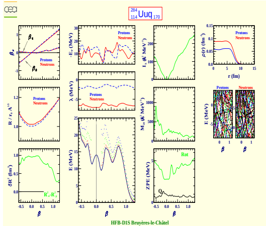
Ununquadium 284 (Z=114, N=170)
