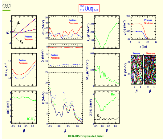
Ununquadium 356 (Z=114, N=242)
