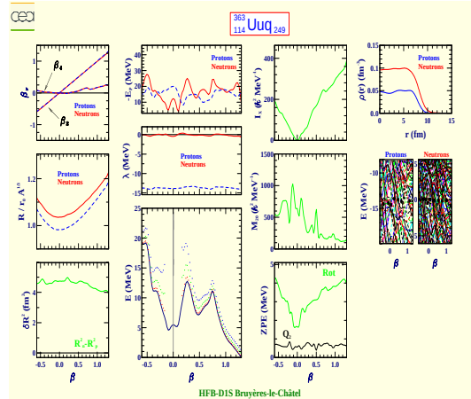
Ununquadium 363 (Z=114, N=249)
