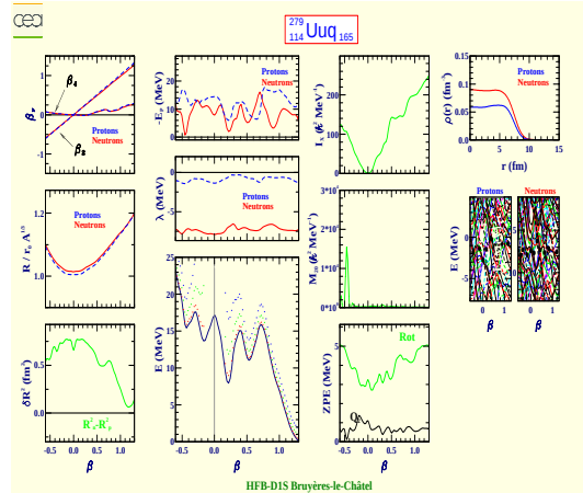
Ununquadium 279 (Z=114, N=165)
