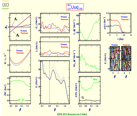
Ununquadium 302 (Z=114, N=188)
