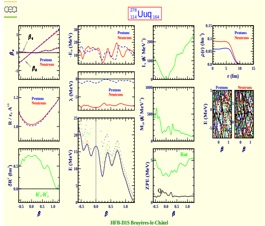
Ununquadium 278 (Z=114, N=164)
