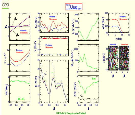
Ununquadium 368 (Z=114, N=254)
