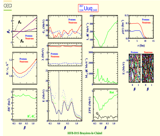
Ununquadium 357 (Z=114, N=243)
