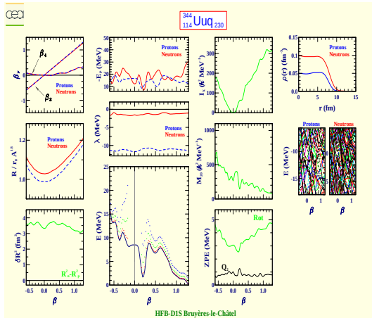
Ununquadium 344 (Z=114, N=230)
