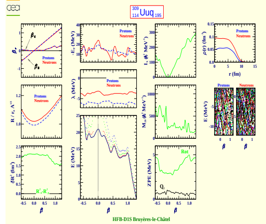
Ununquadium 309 (Z=114, N=195)
