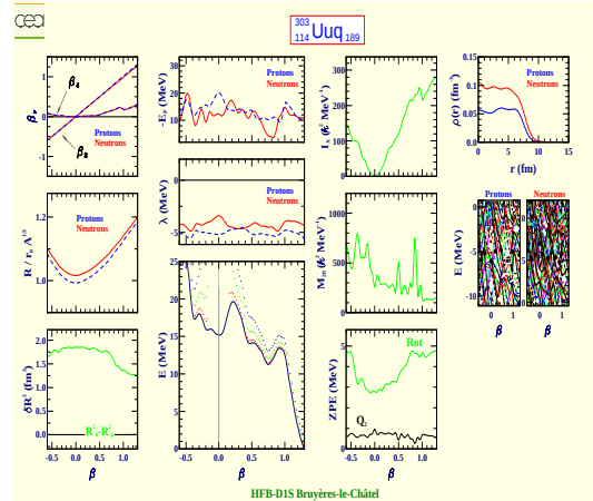
Ununquadium 303 (Z=114, N=189)
