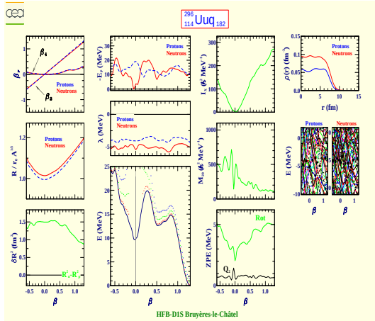
Ununquadium 296 (Z=114, N=182)
