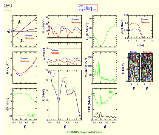
Ununquadium 297 (Z=114, N=183)
