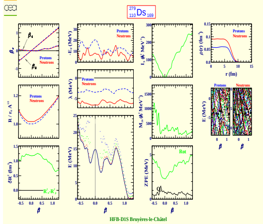
Darmstadtium 279 (Z=110, N=169)
