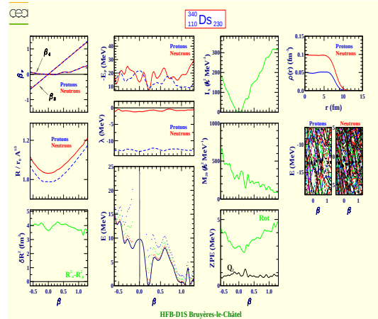
Darmstadtium 340 (Z=110, N=230)
