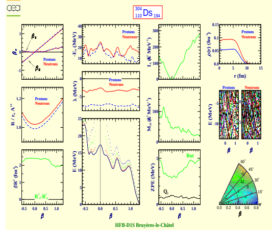
Darmstadtium 304 (Z=110, N=194)
