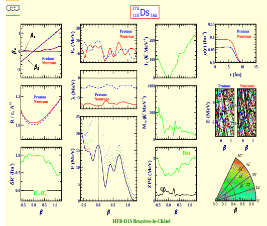
Darmstadtium 274 (Z=110, N=164)
