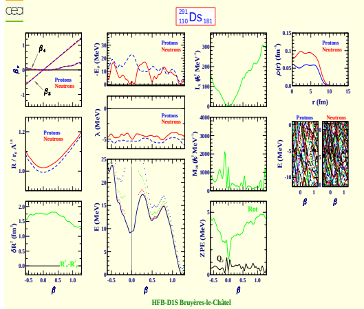
Darmstadtium 291 (Z=110, N=181)
