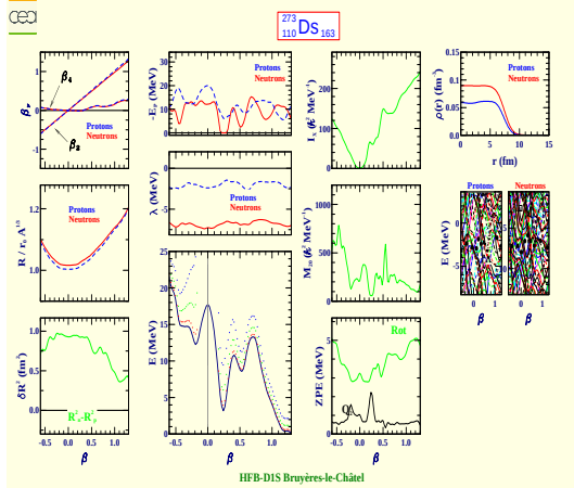
Darmstadtium 273 (Z=110, N=163)
