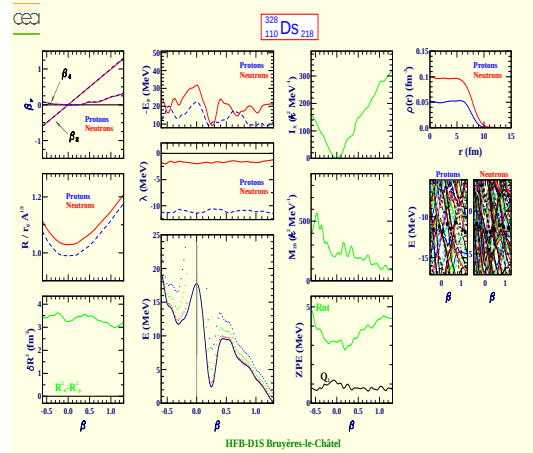
Darmstadtium 328 (Z=110, N=218)
