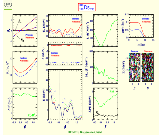
Darmstadtium 346 (Z=110, N=236)
