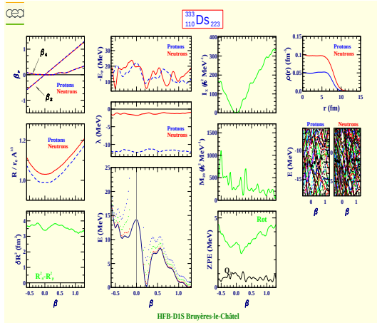
Darmstadtium 333 (Z=110, N=223)
