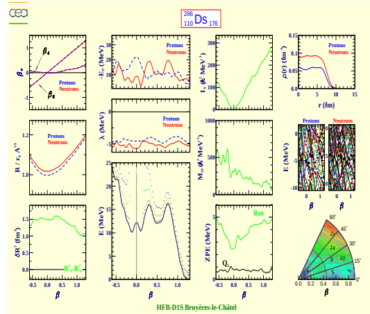
Darmstadtium 286 (Z=110, N=176)
