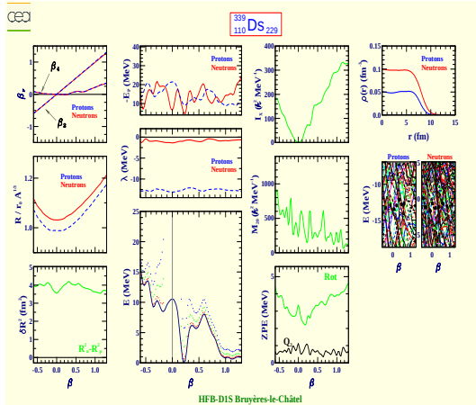
Darmstadtium 339 (Z=110, N=229)
