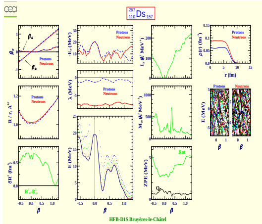
Darmstadtium 267 (Z=110, N=157)
