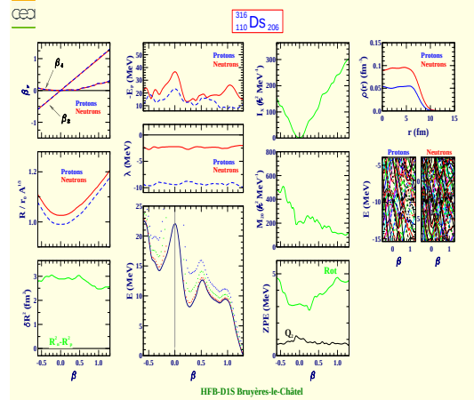
Darmstadtium 316 (Z=110, N=206)
