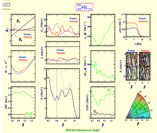
Hassium 284 (Z=108, N=176)
