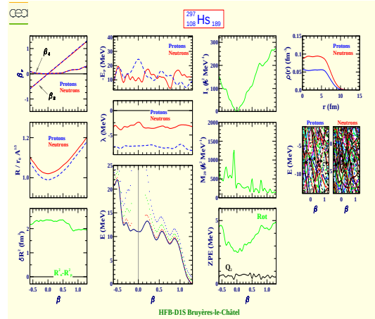
Hassium 297 (Z=108, N=189)
