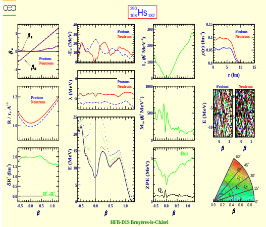
Hassium 290 (Z=108, N=182)
