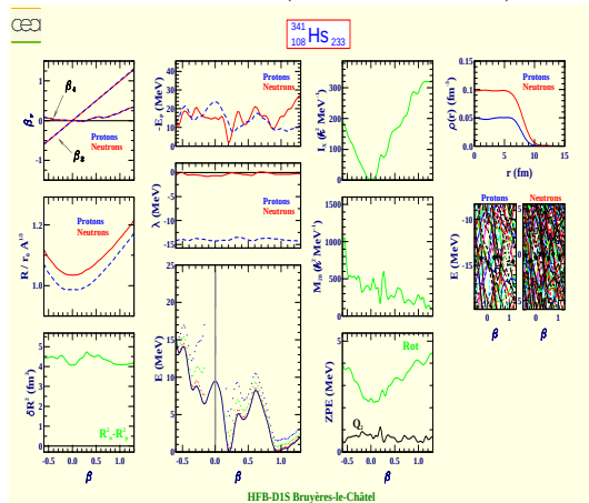
Hassium 341 (Z=108, N=233)
