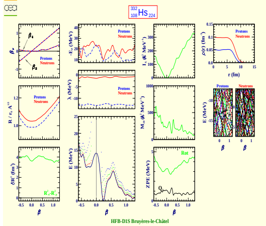
Hassium 332 (Z=108, N=224)
