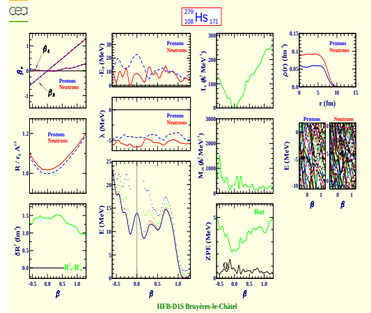
Hassium 279 (Z=108, N=171)
