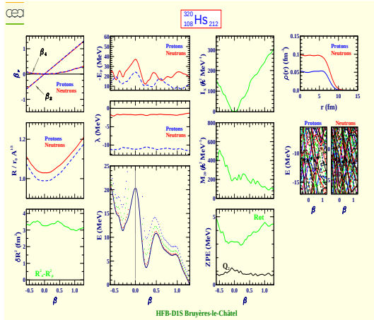
Hassium 320 (Z=108, N=212)
