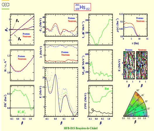
Hassium 260 (Z=108, N=152)
