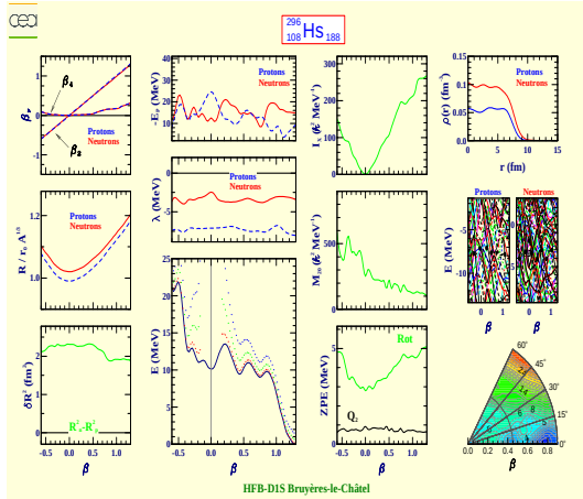
Hassium 296 (Z=108, N=188)
