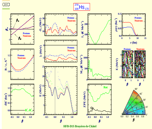
Hassium 278 (Z=108, N=170)
