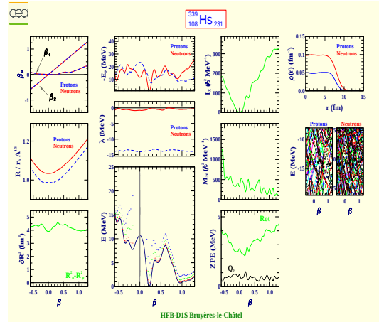
Hassium 339 (Z=108, N=231)
