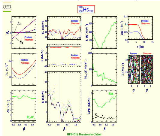
Hassium 340 (Z=108, N=232)
