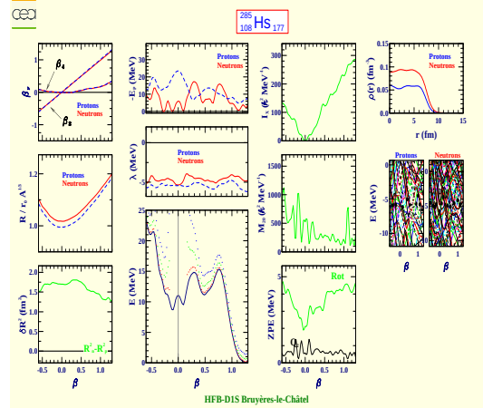
Hassium 285 (Z=108, N=177)
