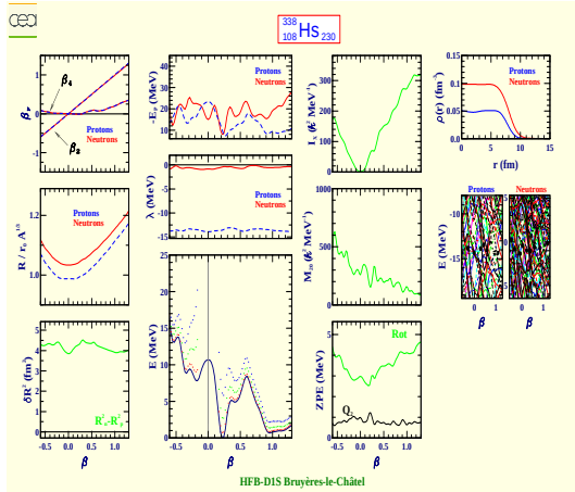
Hassium 338 (Z=108, N=230)
