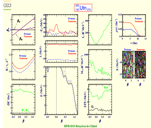
Untrinilium 405 (Z=130, N=275)
